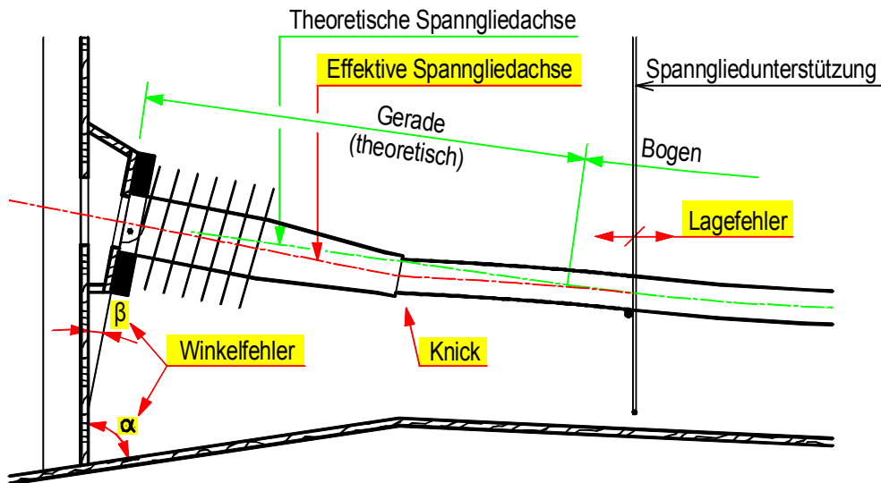
Abb. II.6: Geometrische Randbedingungen.
