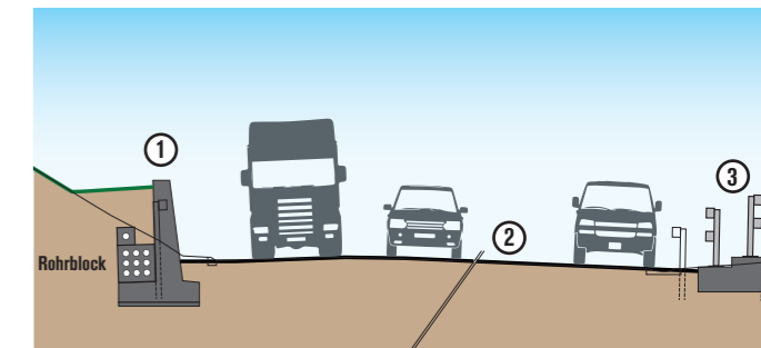
Neue beidseitige Leitmauern ① dichten die Böschungen erneut, aber besser ab. Die Fahrbahn erhält eine neue Deckschicht ②. Beim Mittelstreifen werden Streifenfundamente eingebaut ③.
